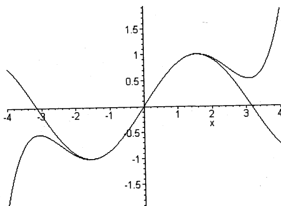
Табл. 12. Приближение синусоиды многочленом
