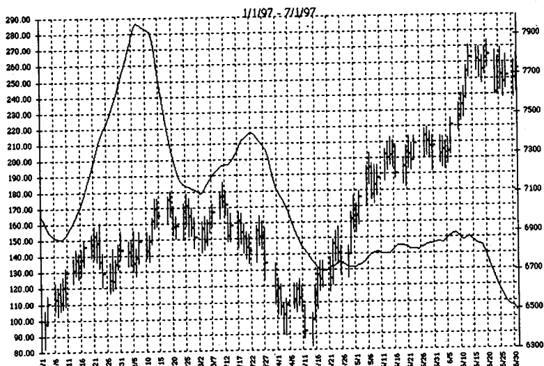
Табл. 10. Сидерограмма Брэдли
