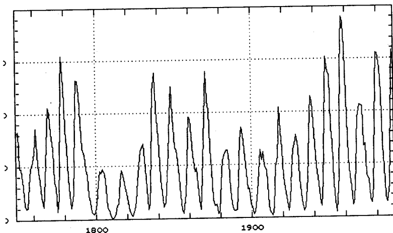
Табл. 11. Динамика чисел Вольфа в 1749-1990 гг.
