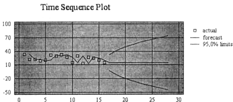
Табл.3. Прогноз по стохастической модели
