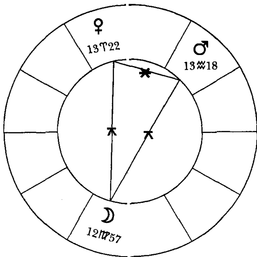
Рис. 23. Йод (Вилы)
